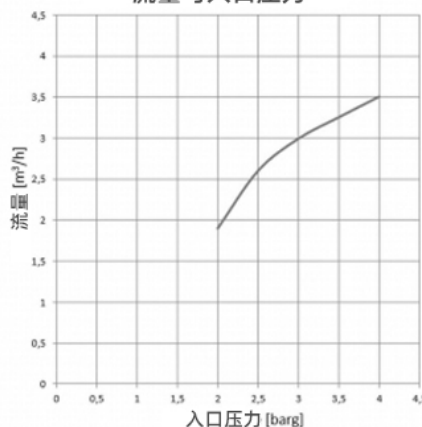
CIP喷嘴低流量 流量与入口压力
